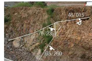
A영역 불연속면 자료
