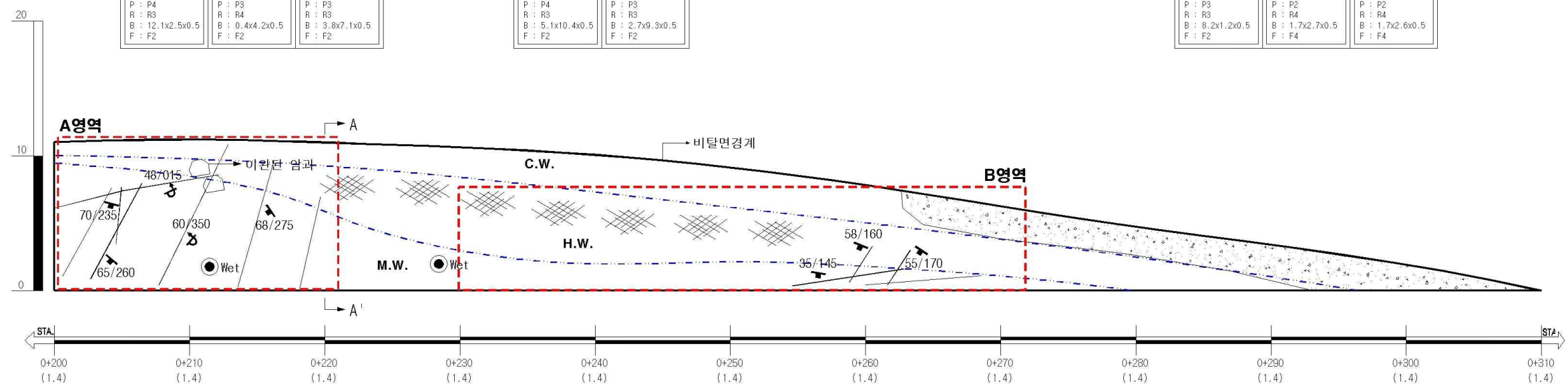
A영역 불연속면 자료
