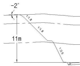
<A-A'단면>
