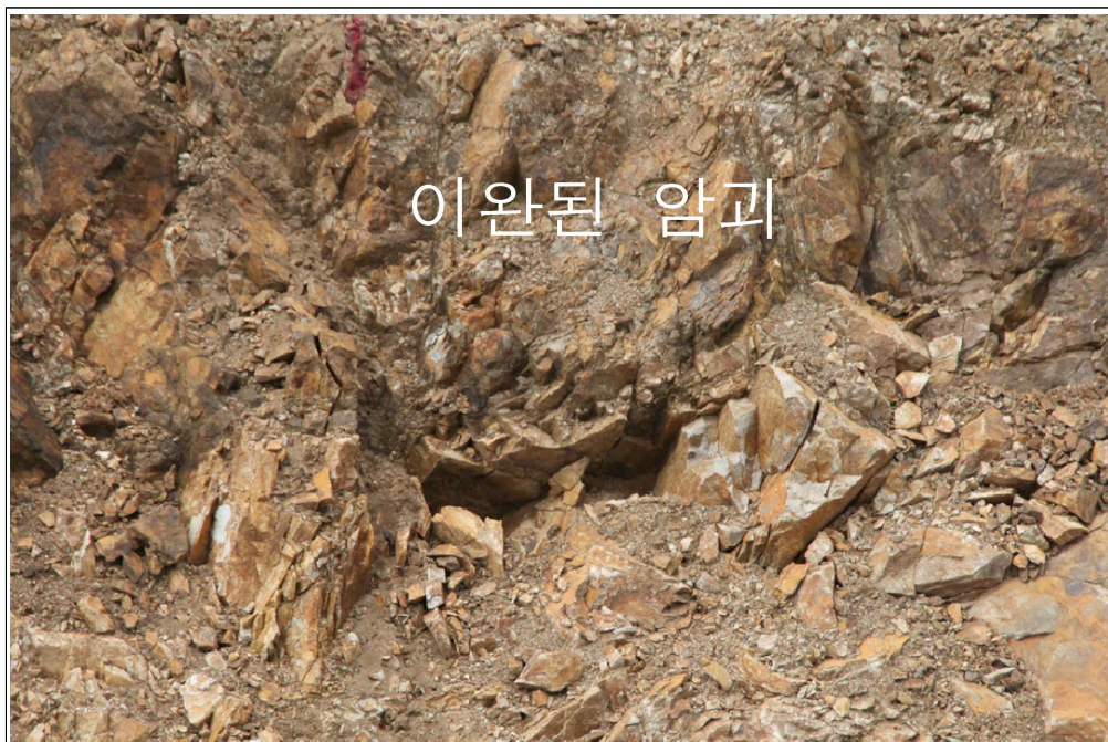
【그림 15】 A 영역 상세사진 (이완된 암괴)
